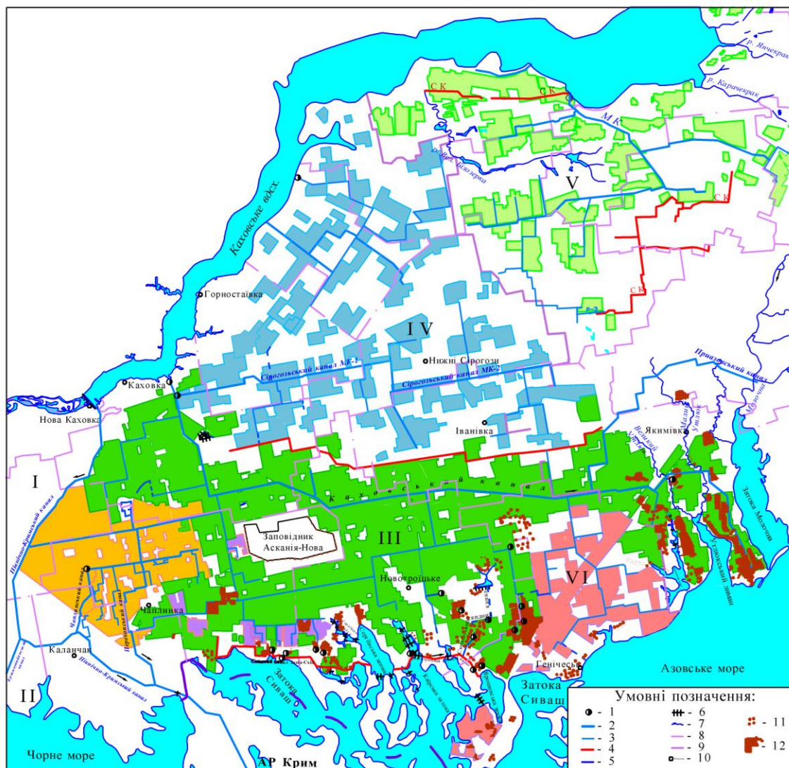
Рисунок 2. Схема зрошення і дренажу на масиві Дніпро - Молочна: I - VI - зрошувальні системи (I - Північно-Кримська, II - Краснознаменська, III - Каховська, IV - Сірогозька, V - Північно-Рогачицька, VI - Генічеська), 1 - насосна станція; 2, 3, 4 - зрошувальні канали; 5 - скидні канали; 6 - греблі; 7 – річка; 8 - границя районів; 9 - границя області; 10 - вертикальний дренаж; 11 - горизонтальний дренаж.
