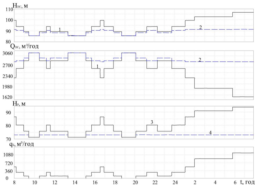
Рисунок 2 - Процеси, що виникають на 33С з БДР при виконанні добового плану-заявки на десять ДМ «Фрегат»
