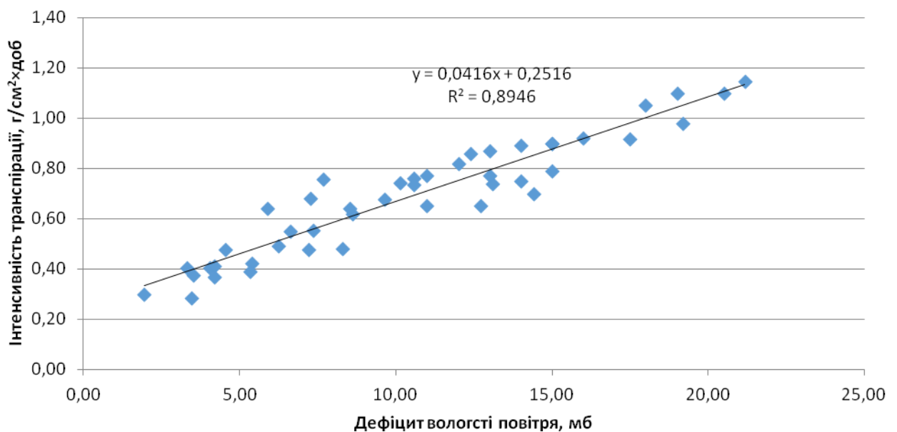
Рисунок 2. Залежність інтенсивності транспірації рослин валеріани лікарської від дефіциту вологості повітря
